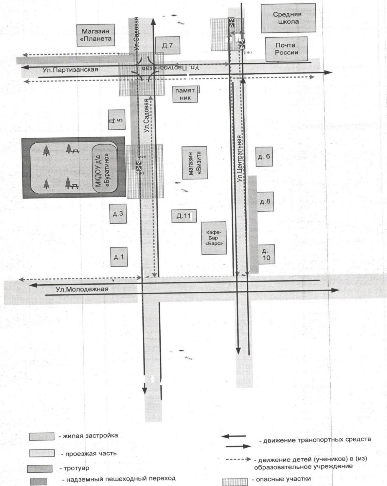
II. Схема организации дорожного движения в непосредственной близости от образовательного учреждения с размещением соответствующих технических средств, маршруты движения детей и расположение парковочных мест
